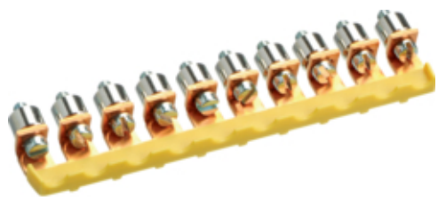
TVERRKOBLING SKRUT 10P 10MM2
