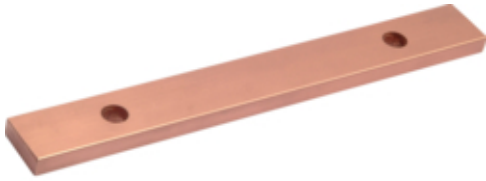
Samleskinne, cu, uN, 30x10x750mm
